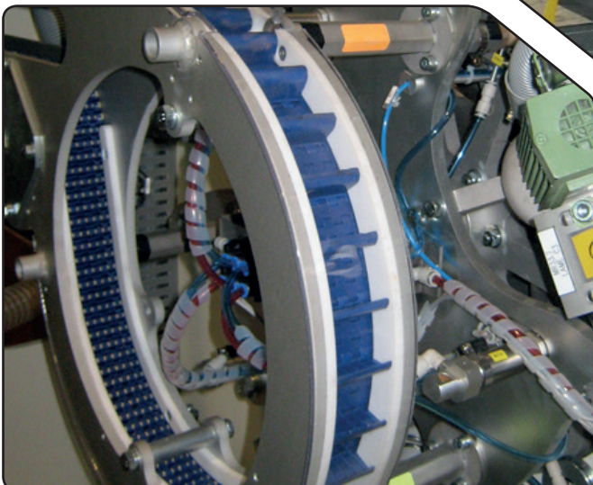
Machine de chanfreinage de bouchons (Belgique)
