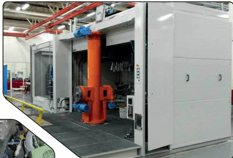
Banc de test de valves hydrauliques (Belgique)
