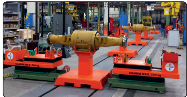
Ligne de montage d'essieux (Belgique)
