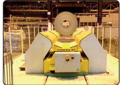
Navette à induction (France)
